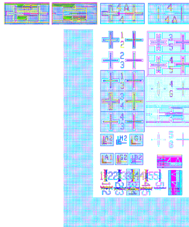
Bild 3: Positioniermarken und Vernierelemente zur Feinpositionierung der einzelnen Lithographieebenen, sowie großes L zum Groben Ausrichten.
