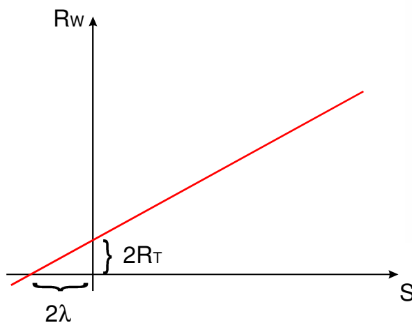
Bild 11: Ermittlung des Kontaktwiderstandes R_T und der Transferlänge \lambda .
