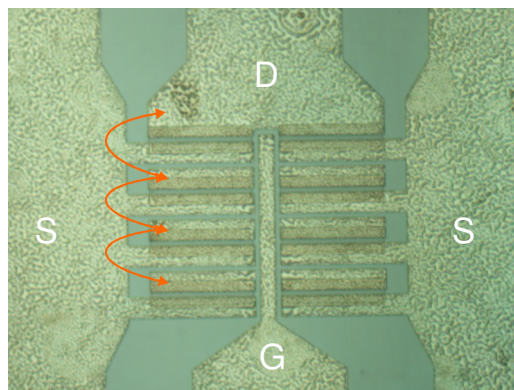
Bild 13: Struktur eines Multifinger-Transistors nach der Metallisierung der ohmschen Kontakte. Bezeichnet sind Source (S), Drain (D) und Gate (G); die Pfeile verdeutlichen die zu definierenden Luftbrücken zur Herstellung der Drainverbindungen.
