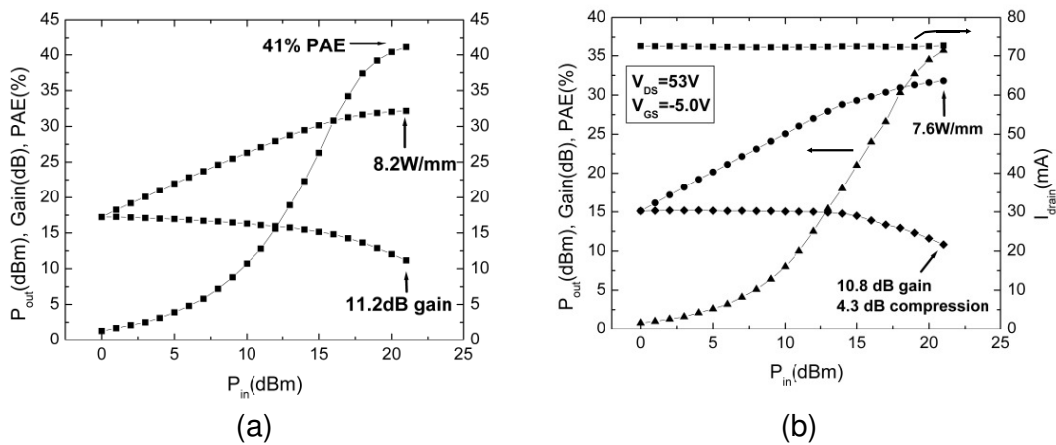
Bild 21: Load-Pull-Messungen bei 2 GHz an HEMTs mit einer Peripherie von 200 \mu\text{m} und Gatelängen von 1 \mu\text{m} (a) und 2 \mu\text{m} (b). Am Bauelement in Bild (a) wurde ein Arbeitspunkt von V_{DS} = 45\text{ V} und V_{GS} = -4,7\text{ V} eingestellt, wobei eine Leistungsdichte von 8,2 W/mm ermittelt wurde. Die Effizienz beträgt 41%. Exemplarisch zeigt Bild (b) das Verhalten eines 1 \mu\text{m} -Transistors mit vernachlässigbarem Drainstromkollaps.
