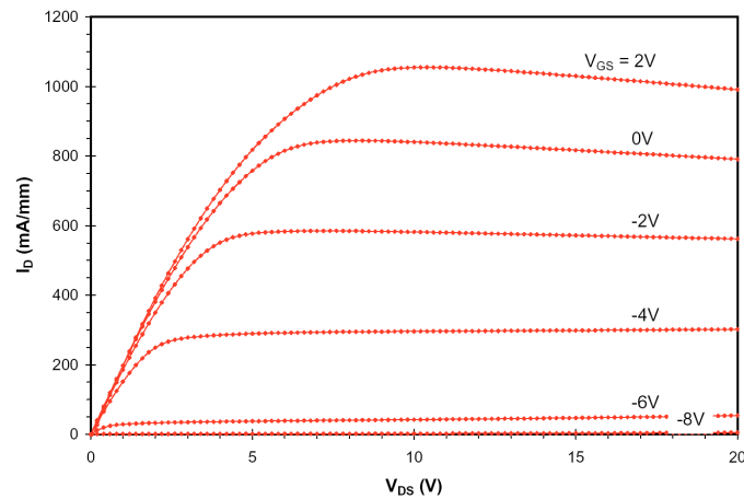
Bild 17: Ausgangskennlinien für ein Bauelement mit einer Gatelänge von 2\ \mu\text{m} , einer Peripherie von 150\ \mu\text{m} und einem Drain-Source-Abstand von 6\ \mu\text{m} . Der maximale Drainstrom beträgt 1055\ \text{mA/mm} .
