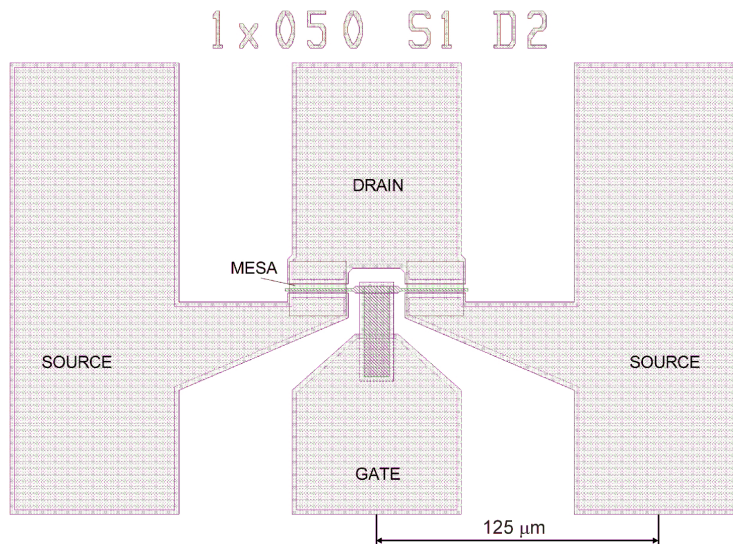
Bild 4: Layout eines Doppelgate-HEMTs mit 1\ \mu\text{m} Gatelänge und einer Gatebreite von 2 \times 25\ \mu\text{m} . Das Rastermaß zwischen Drain und Source bzw. Drain und Gate beträgt 125\ \mu\text{m} . Der Gate-Source Abstand beträgt 1\ \mu\text{m} , die Distanz des Gates zum Drain 2\ \mu\text{m} . Bezeichnet sind die Kontaktflächen von Drain, Source und Gate. Die eigentliche Gateebene wird durch das grün schraffierte Gebiet symbolisiert.
