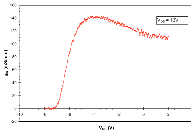
Bild 18: Steilheit g_m für dasselbe 150\ \mu\text{m} -Bauelement wie in Bild 17, gemessen bei einer Drain-Source-Spannung von 13\ \text{V} .
