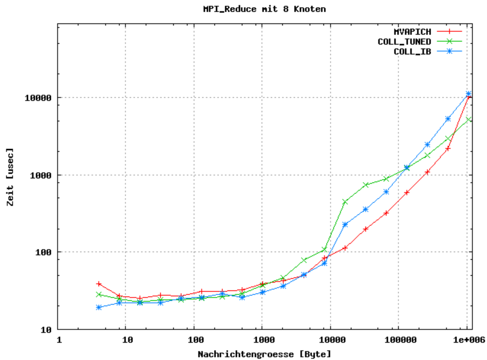
Bild 29. MPI_Reduce() mit 8 Knoten
