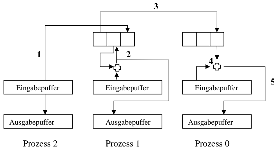
Bild 28. Ablauf des Pipeline-Prinzips bei MPI_Scan am Beispiel von 3 Prozessoren
